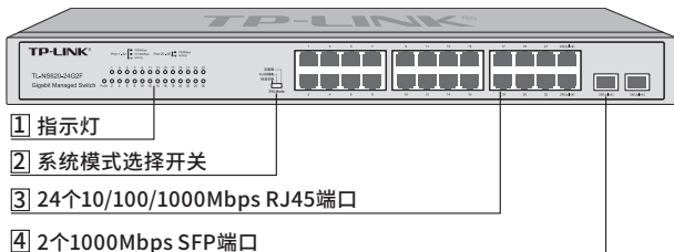
图1-2 TL-NS620-24G2F前面板示意图
