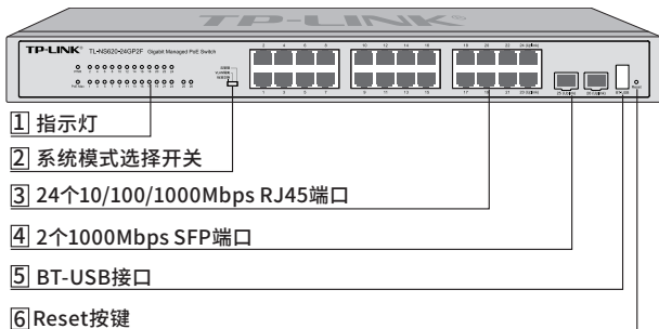
图1-3 TL-NS620-24GP2F前面板示意图
