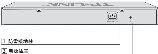
图1-6 TL-NS620-24GP2F后面板示意图
