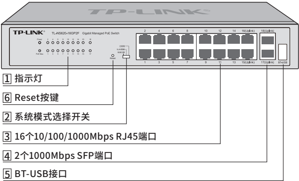
图1-4 TL-NS620-16GP2F前面板示意图
